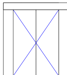
imposte partie fixe latérale panneau plein ou vitrée
