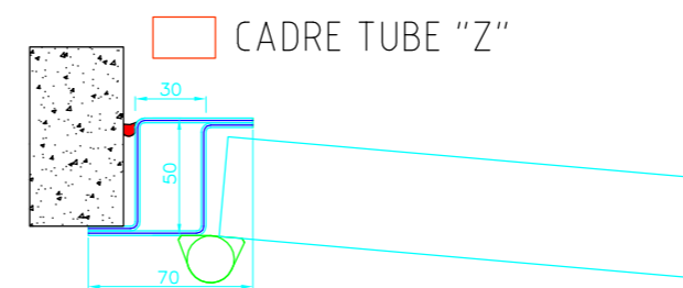
COUPE IMPOSTE
