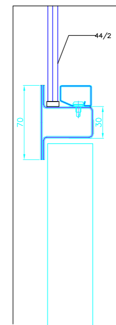
COUPE IMPOSTE
