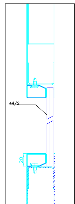
COUPE OCULUS
