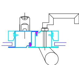
GACHE ELCTRIQUE + SERR 1Pt BEQUILLE INT. BATON EXT CREMONE POMPIER
