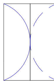
Porte 2 vantaux sur pivots va-et-vient anti-pince doigts
