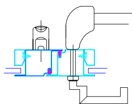
ANTIPANIQUE MODULE EXTERIEUR CREMONE POMPIER
