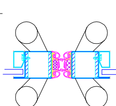
VERSION VA ET VIENT BATON DE MARECHAL
