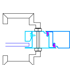
SERRURE 1 POINT PENE 1/2 T SELON PV BEQUILLE DOUBLE
