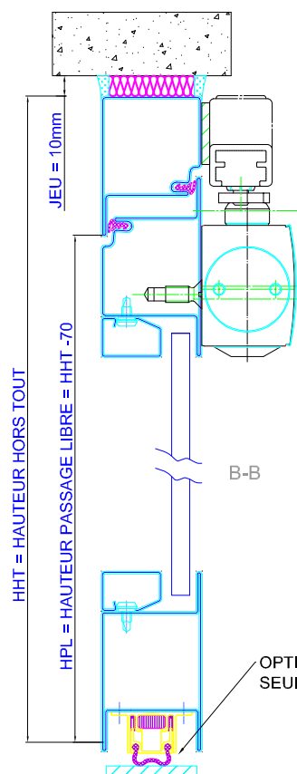
SERRURE 1 POINT PENE 1/2 T SELON PV BEQUILLE DOUBLE
