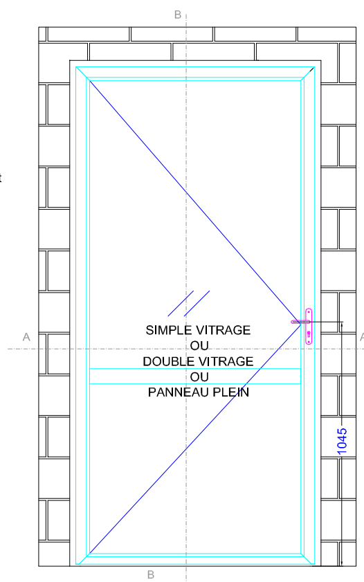
OPTION Porte DAS - NFS 61 937 MODE 2 normalement ouvert
