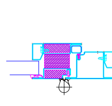
INTEGRATION DANS CHASSIS COUPE FEU NOFEU EI30 NOFEU EI60
