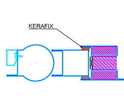
INTegration DANS CHASSIS COUPE FEU NOFEU EI60
