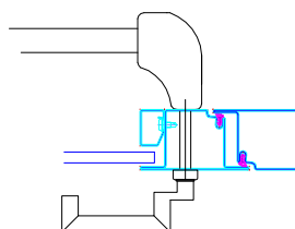
SERRURE ANTIPANIQUE 1 PT OU 2 PTS SELON PV MODULE EXTERIEUR
