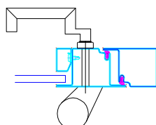
GACHE ELECTRIQUE SERRURE 1 PT BEQUILLE INT. BATON EXT
