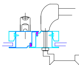
ANTIPANIQUE MODULE EXTERIEUR CREMONE POMPIER
