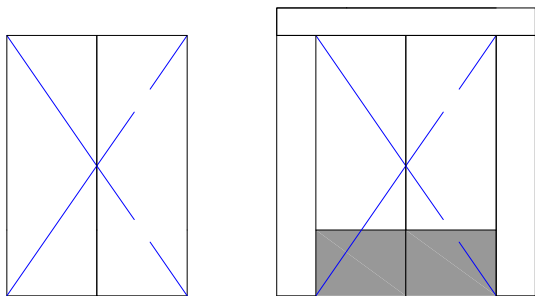
Porte 2 vantaux, avec ou sans imposte, avec ou sans partie fixe latérale avec et sans parties pleines
