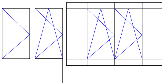
Ouvrants de Service E30 uniquement A frappe ou Oscillot Battant avec ou sans imposte, avec ou sans allège avec ou sans partie fixe latérale
