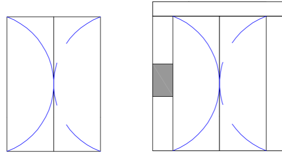
Porte 2 vantaux sur pivots va-et-vient anti-pince doigts imposte partie fixe latérale panneau plein cintrage poteau technique
