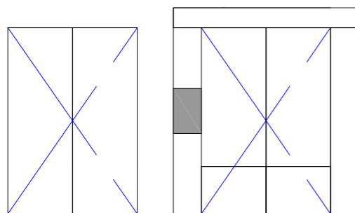
Porte 2 vantaux, sur paumelles imposte partie fixe latérale panneau plein cintrage poteau technique
