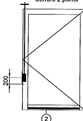
Vantail hauteur maxl 2256 Serrure 2 points
