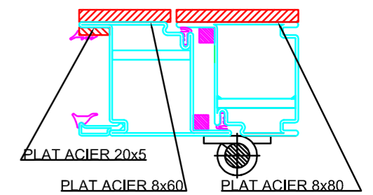
PROFIL FB6
