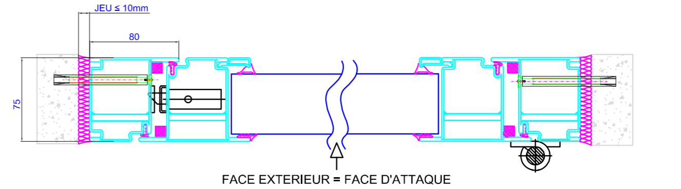
PROFIL FB6
