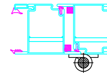
PROFIL FB4
