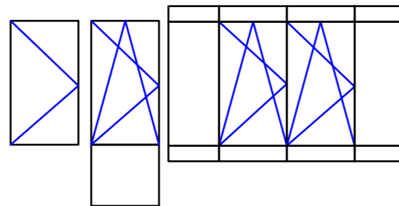
Fenêtre 1 Vantail A frappe ou Oscillot Battant avec ou sans imposte, avec ou sans allège avec ou sans partie fixe latérale
