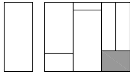
Châssis fixe et baie vitrée imposte partie fixe latérale panneau plein allège
